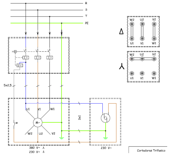
Cartadoras Trifásico
