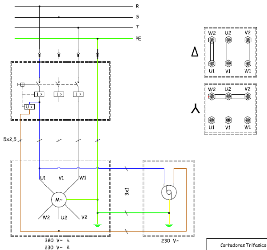
Cartadoras Trifásico
